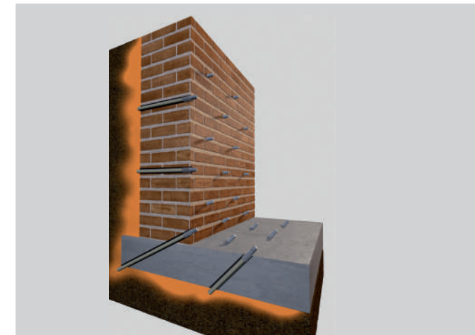
Beispiel: Schleierinjektion
